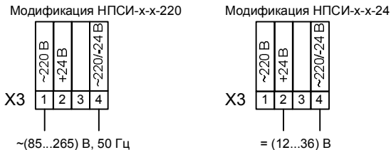
Рисунок 7г – Подключение питания
